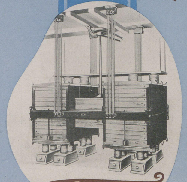
4teiliger-Plansichter
